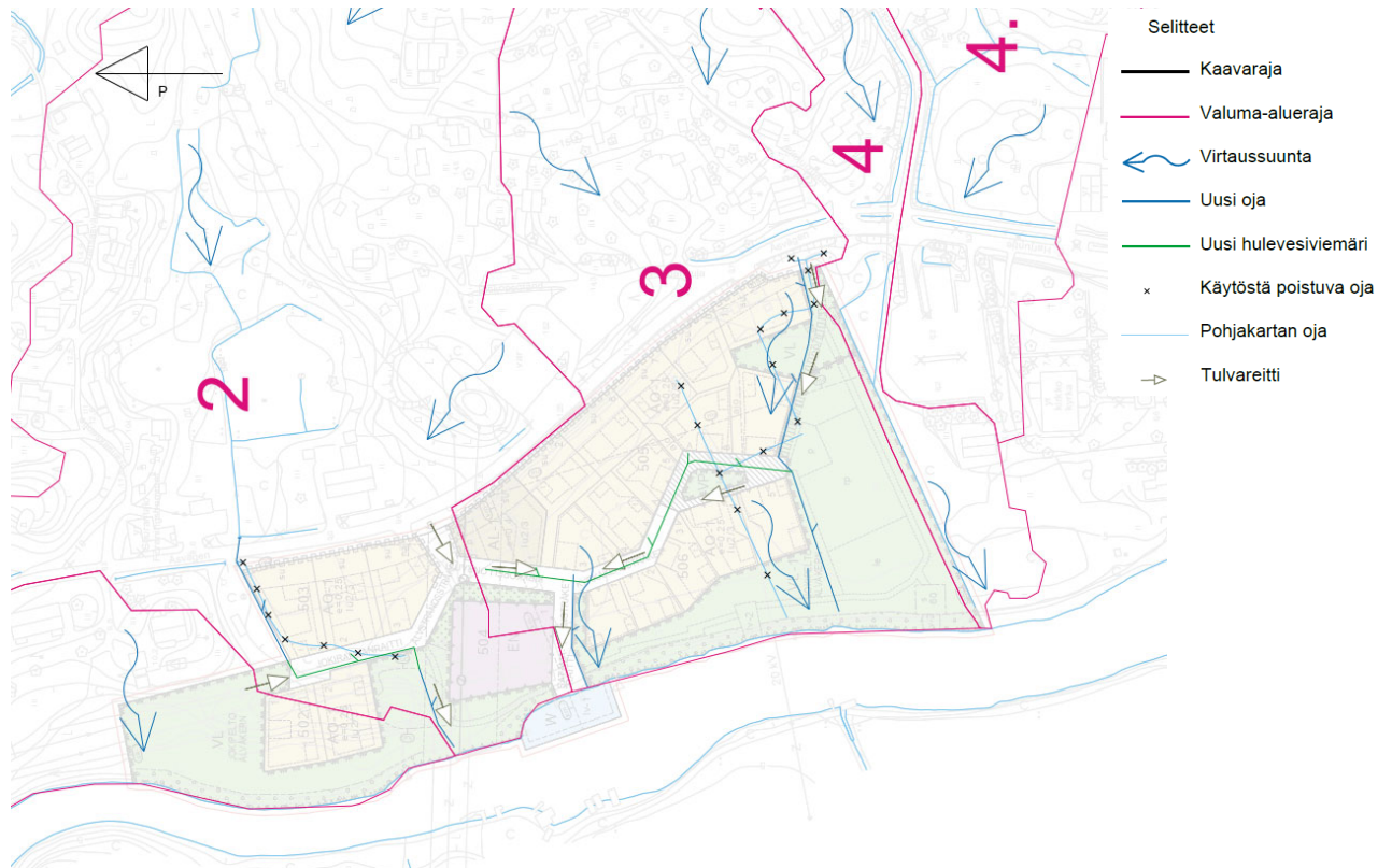
Kuva 4. Suunnittelualueen osavaluma-alueet ja virtaussuunnat.
