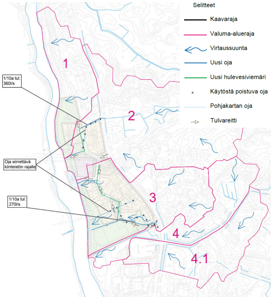
Kuva 5. Uudet ja poistuvat virtausreitit.
