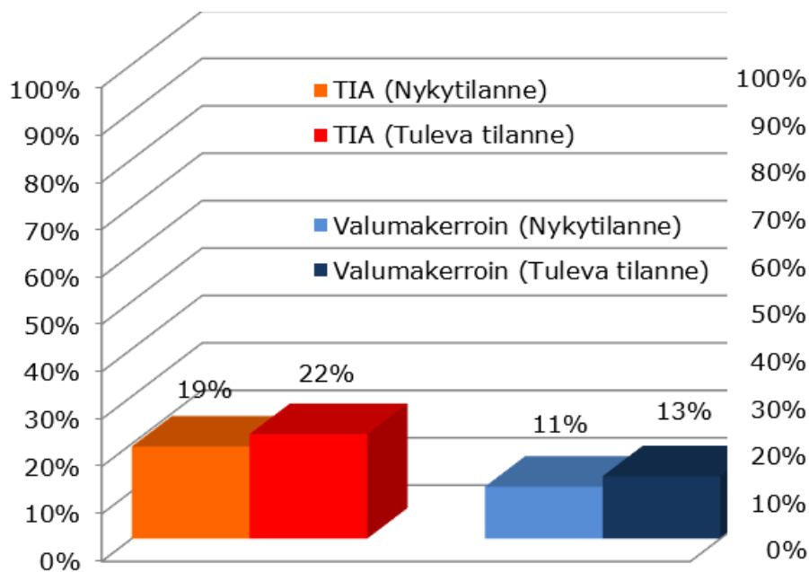
Kuva 6. Osavaluma-alueiden maankäytön aiheuttamat muutokset läpäisemättömän pinnan osuuteen alueen pinta-alasta (TIA) sekä valumakertoimeen (määritetty sadetapahtumalle Tn. 5 kesto 15 min).
