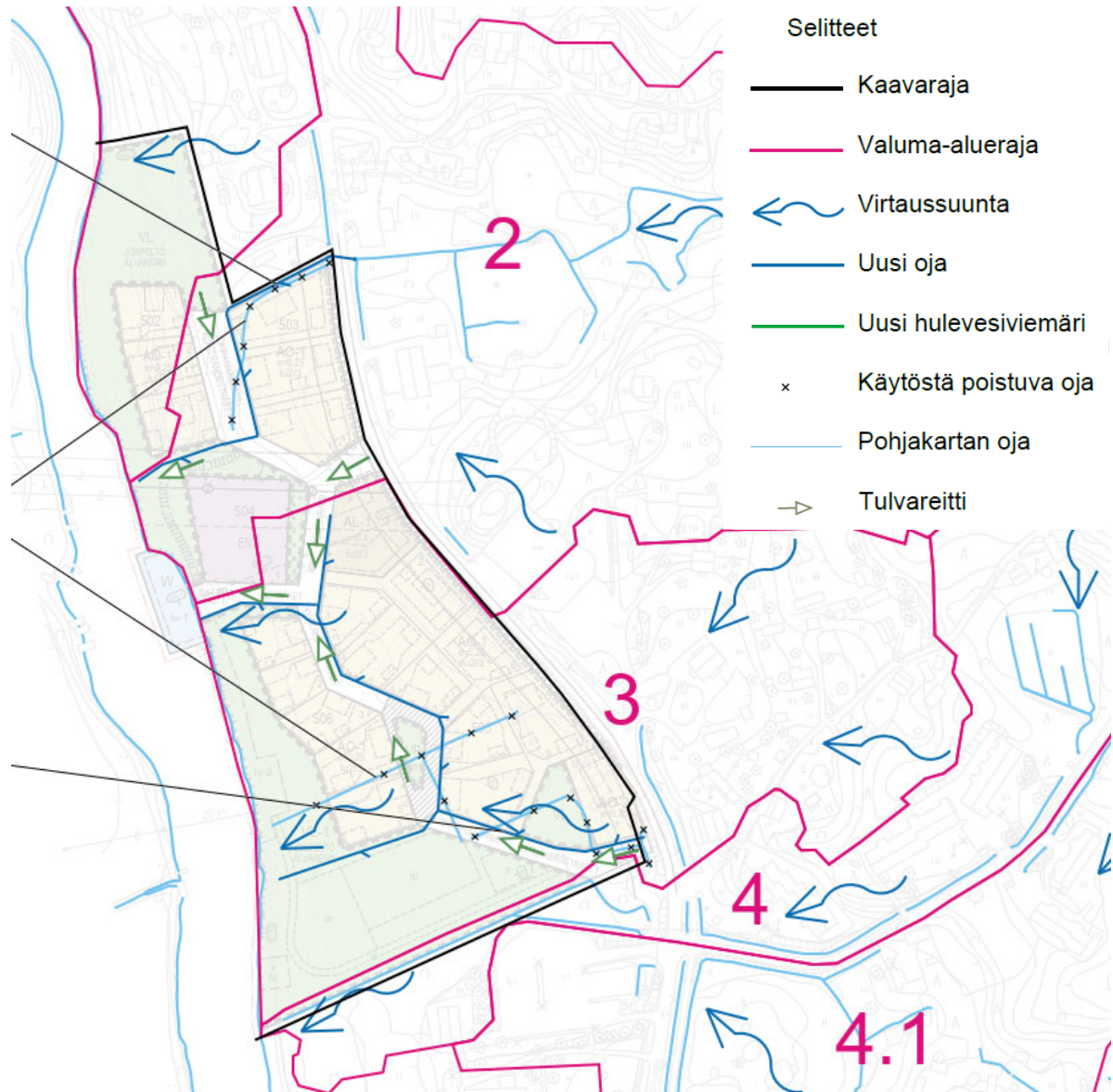
Kuva 7. Tulvareitit merkattu karttaan vihreillä nuolilla
