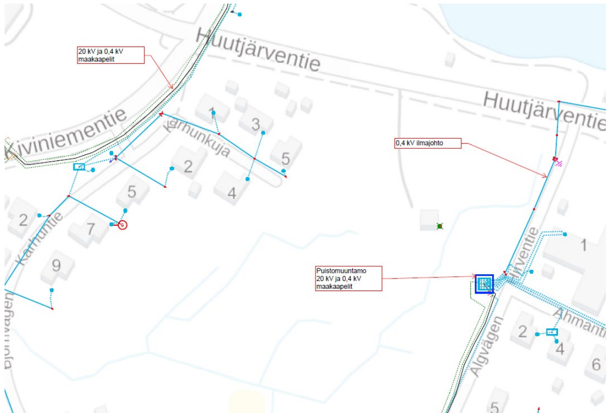
Kuva 1. Ote lausunnon liitteestä, jossa on kuvattu alueen sähköverkko.
